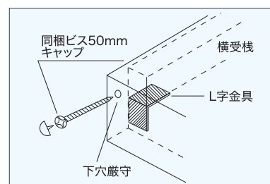
大壁中棚
