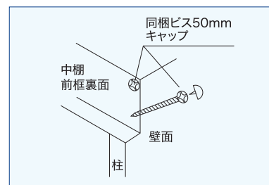
真壁中棚
