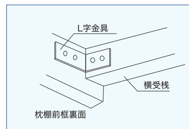
枕棚
